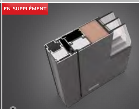
Profilé CarbonCore avec isolation supplémentaire
